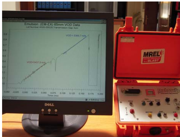
Μέτρηση ταχύτητας έκρηξης με MicroTrap VOD Data Recorder
